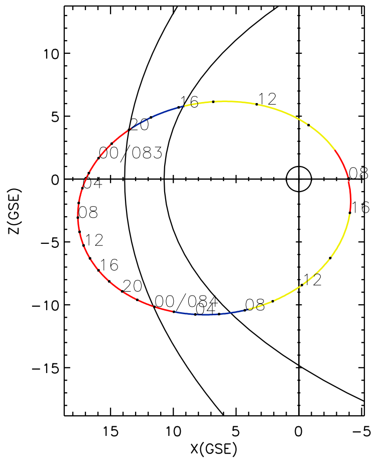
CLUSTER 2 orbit 2005 082 (03/23) 07:56 UT to 2005 084 (03/25) 17:01 UT
