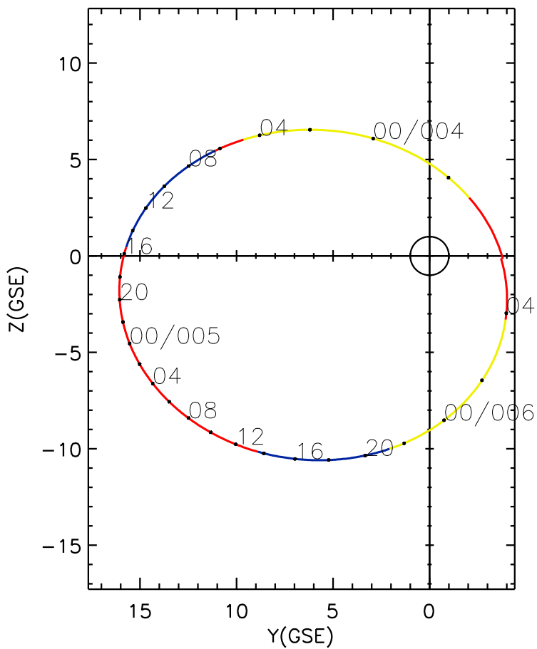
CLUSTER 2 orbit 2005 003 (01/03) 20:06 UT to 2005 006 (01/06) 05:11 UT
