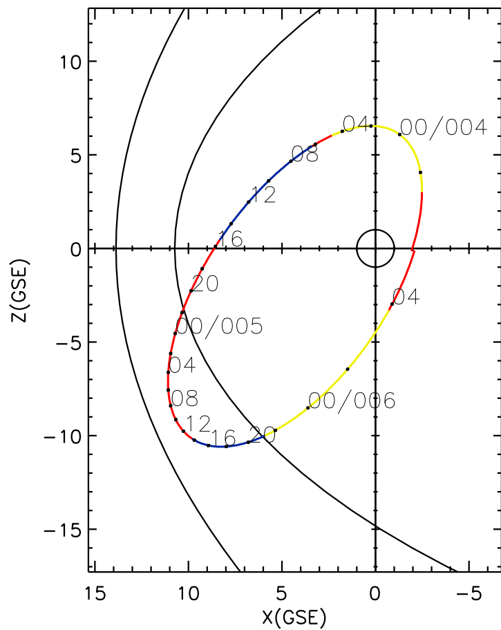
CLUSTER 2 orbit 2005 003 (01/03) 20:06 UT to 2005 006 (01/06) 05:11 UT
