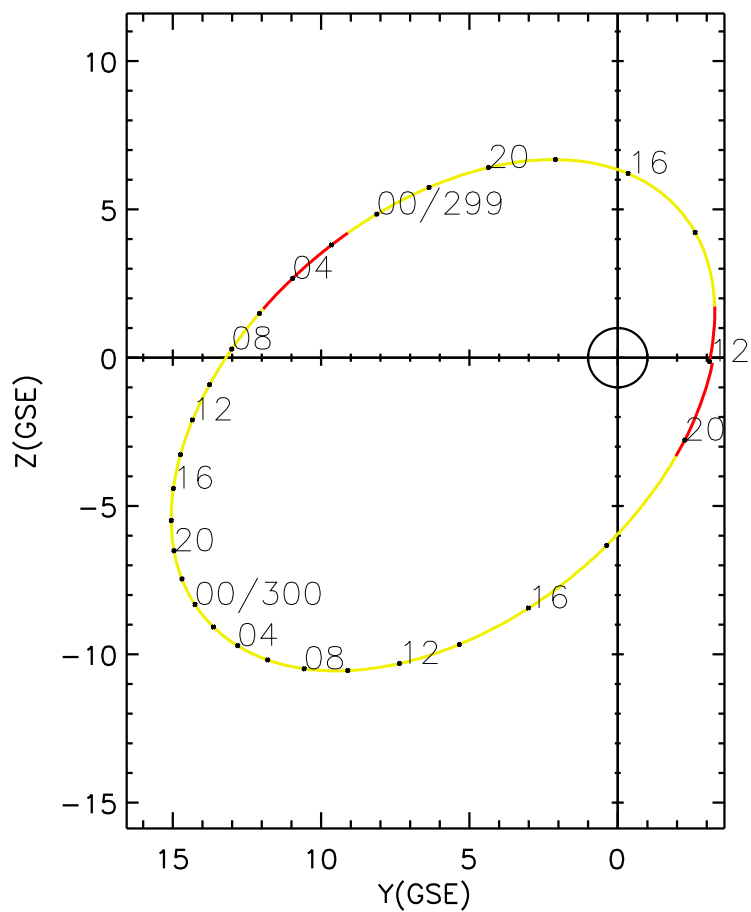
CLUSTER 2 orbit 2004 298 (10/24) 12:00 UT to 2004 300 (10/26) 21:05 UT
