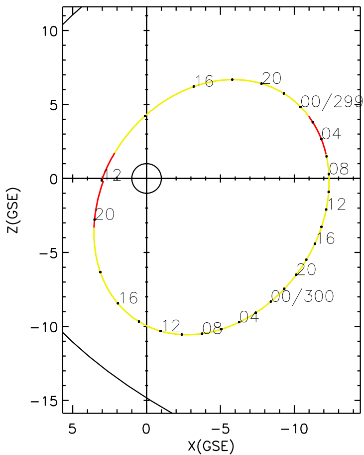
CLUSTER 2 orbit 2004 298 (10/24) 12:00 UT to 2004 300 (10/26) 21:05 UT
