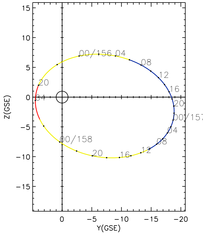
CLUSTER 2 orbit 2004 155 (06/03) 19:06 UT to 2004 158 (06/06) 04:11 UT
