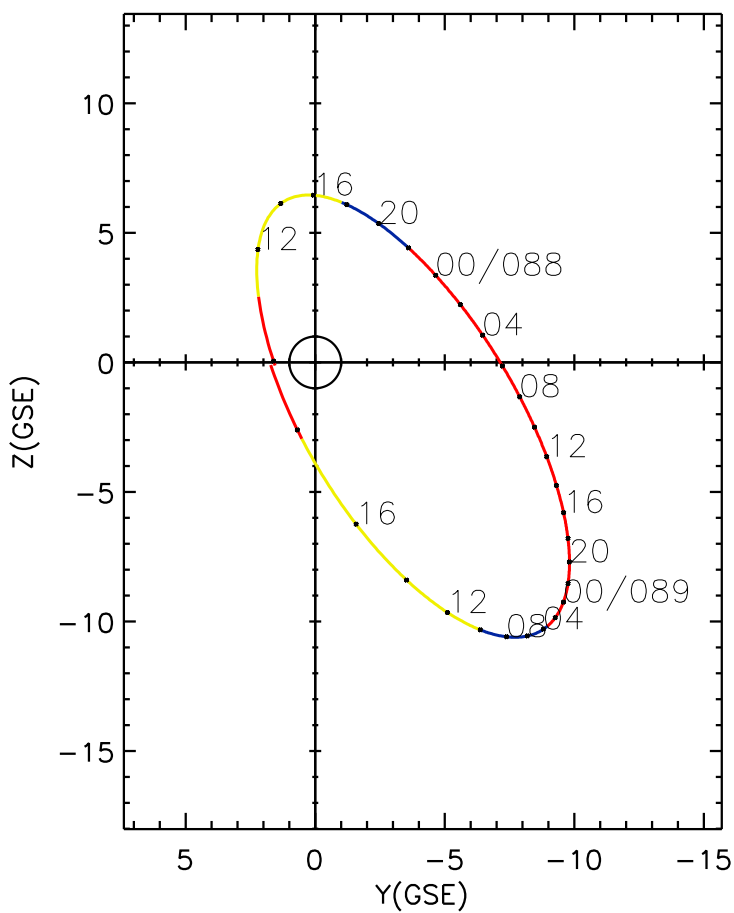
CLUSTER 2 orbit 2004 087 (03/27) 09:56 UT to 2004 089 (03/29) 19:01 UT
