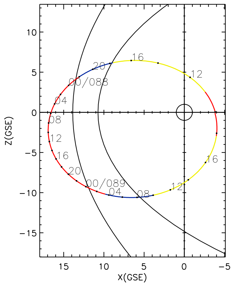
CLUSTER 2 orbit 2004 087 (03/27) 09:56 UT to 2004 089 (03/29) 19:01 UT
