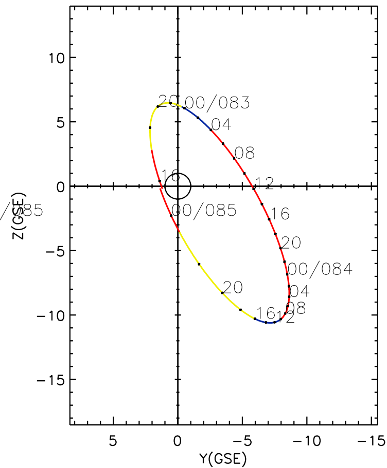
CLUSTER 2 orbit 2004 082 (03/22) 15:46 UT to 2004 085 (03/25) 00:51 UT
