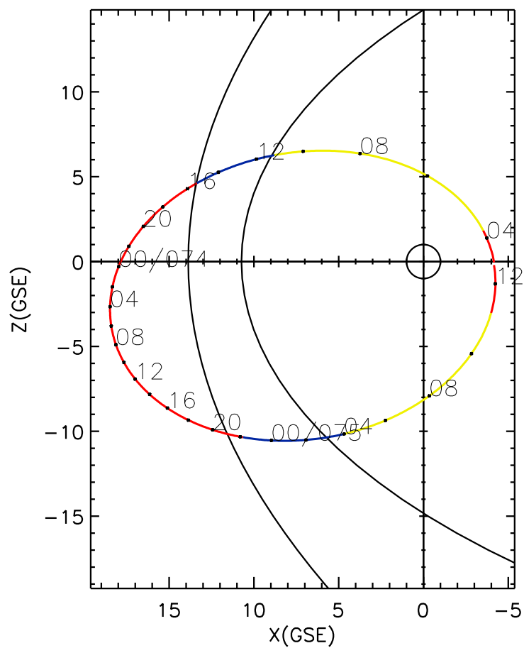
CLUSTER 2 orbit 2004 073 (03/13) 03:26 UT to 2004 075 (03/15) 12:26 UT
