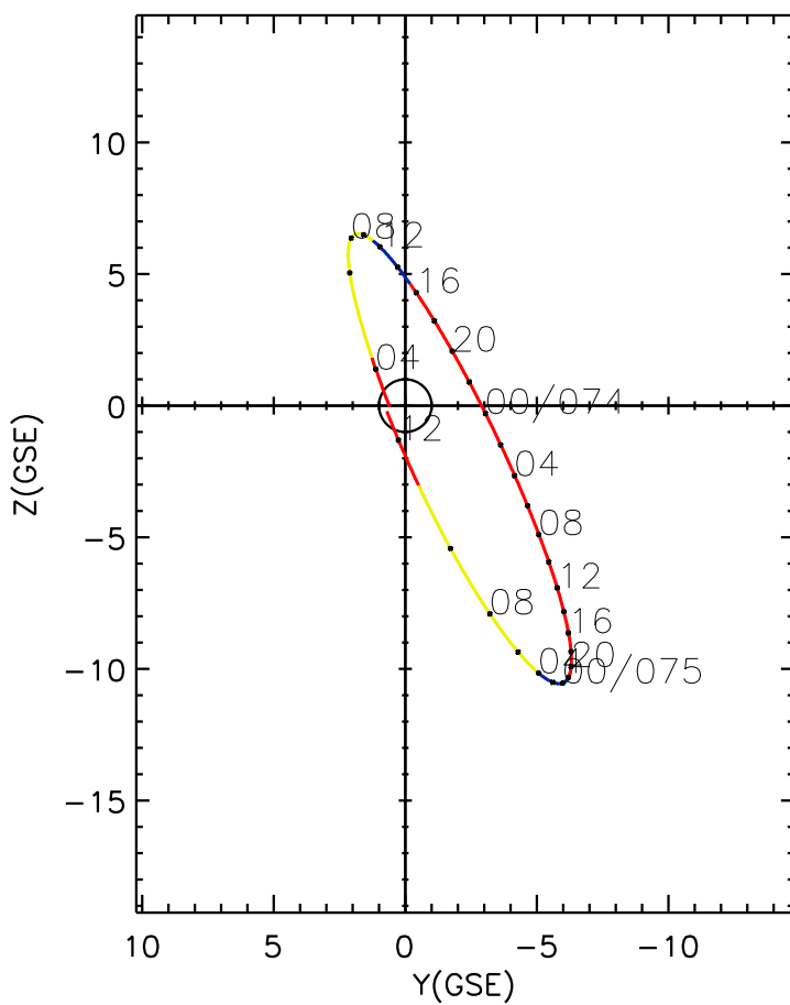
CLUSTER 2 orbit 2004 073 (03/13) 03:26 UT to 2004 075 (03/15) 12:26 UT
