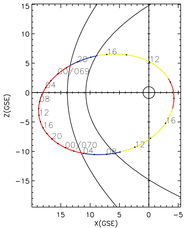
CLUSTER 2 orbit 2004 068 (03/08) 09:16 UT to 2004 070 (03/10) 18:21 UT
