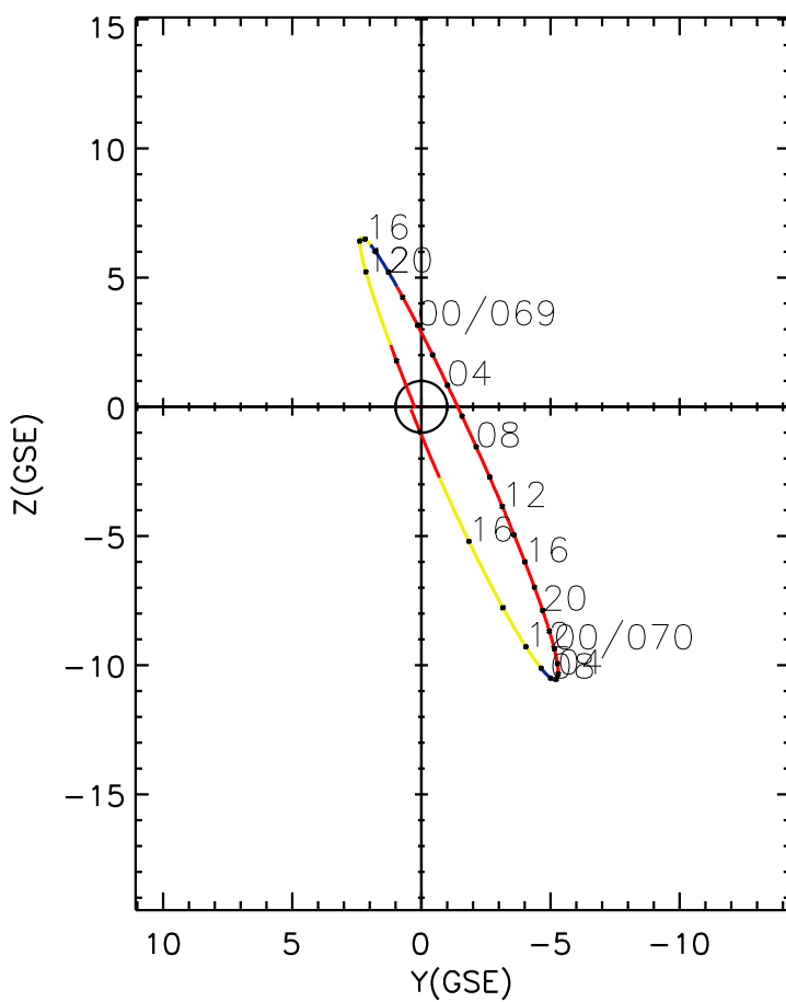
CLUSTER 2 orbit 2004 068 (03/08) 09:16 UT to 2004 070 (03/10) 18:21 UT
