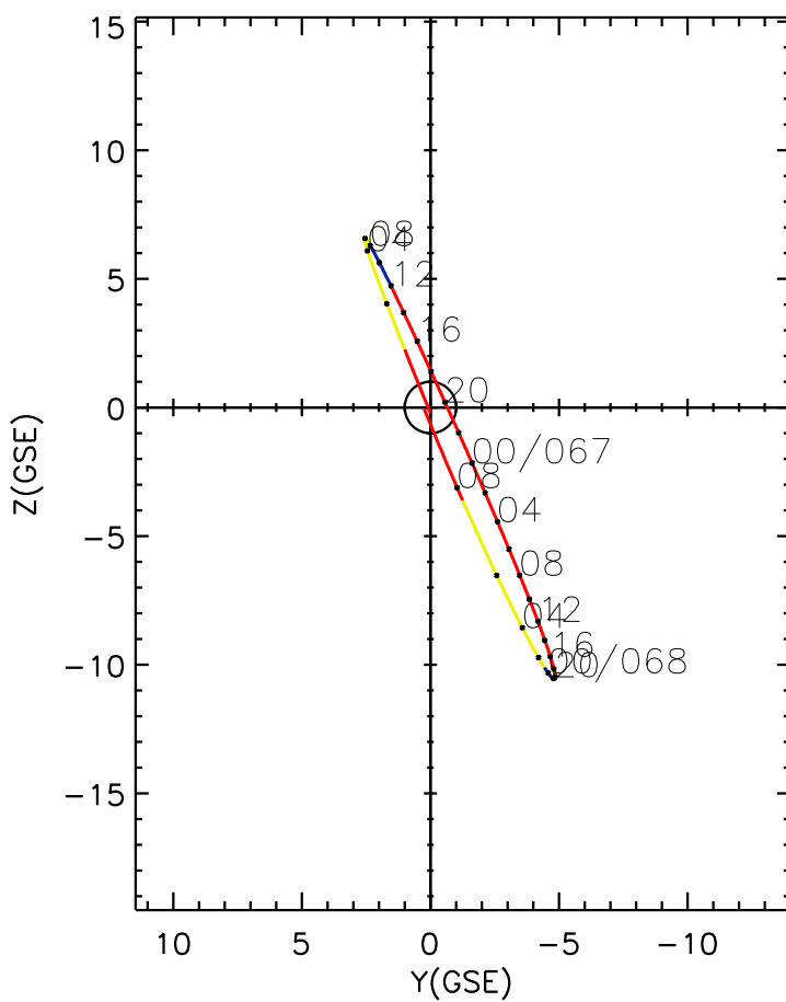
CLUSTER 2 orbit 2004 066 (03/06) 00:06 UT to 2004 068 (03/08) 09:16 UT
