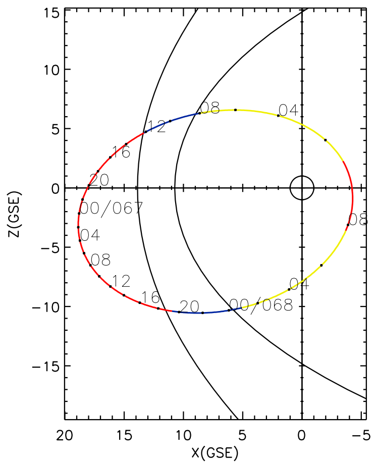
CLUSTER 2 orbit 2004 066 (03/06) 00:06 UT to 2004 068 (03/08) 09:16 UT
