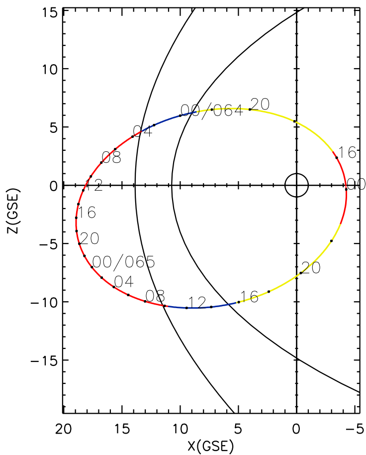
CLUSTER 2 orbit 2004 063 (03/03) 15:00 UT to 2004 066 (03/06) 00:05 UT
