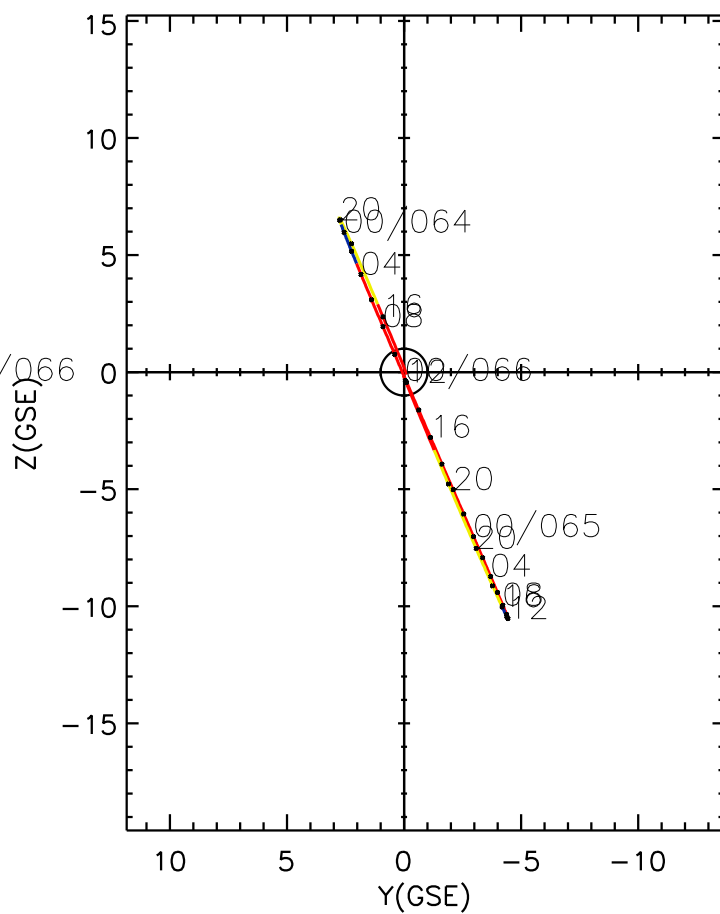
CLUSTER 2 orbit 2004 063 (03/03) 15:00 UT to 2004 066 (03/06) 00:05 UT
