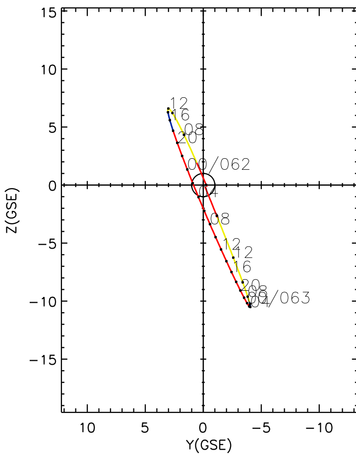
CLUSTER 2 orbit 2004 061 (03/01) 05:56 UT to 2004 063 (03/03) 15:01 UT
