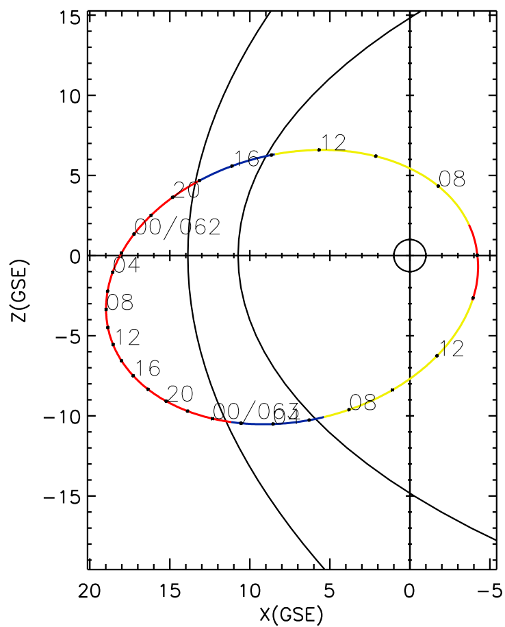
CLUSTER 2 orbit 2004 061 (03/01) 05:56 UT to 2004 063 (03/03) 15:01 UT
