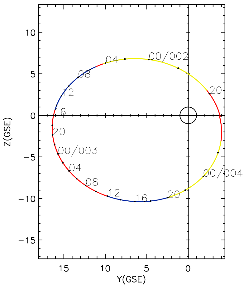
CLUSTER 2 orbit 2004 001 (01/01) 18:51 UT to 2004 004 (01/04) 03:56 UT
