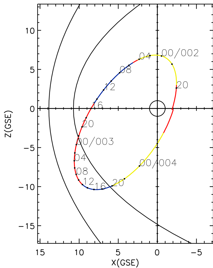
CLUSTER 2 orbit 2004 001 (01/01) 18:51 UT to 2004 004 (01/04) 03:56 UT
