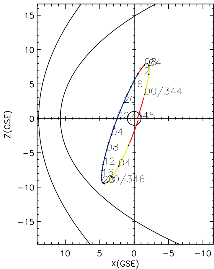
CLUSTER 2 orbit 2002 343 (12/09) 22:30 UT to 2002 346 (12/12) 07:35 UT
