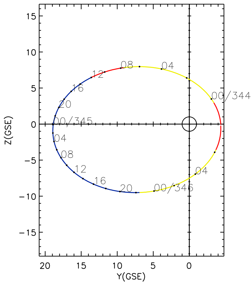
CLUSTER 2 orbit 2002 343 (12/09) 22:30 UT to 2002 346 (12/12) 07:35 UT
